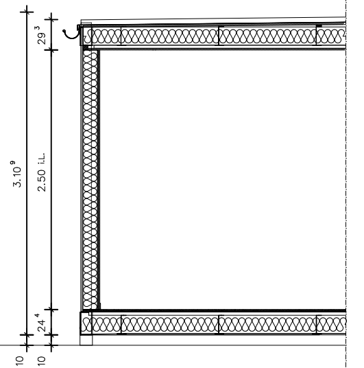
Schnitt A-A M 1:50
